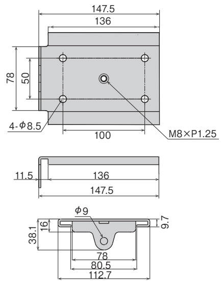
●コードマックL、XL用 (CLD、CXD型)
