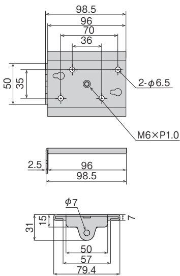
●コードマックS、MS用 (CSS、CBS型)
