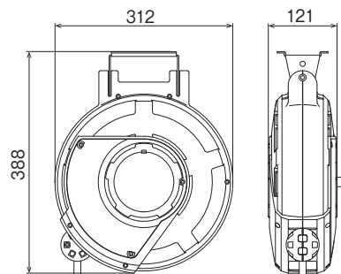
コードマックⅡ CDSⅡ型
