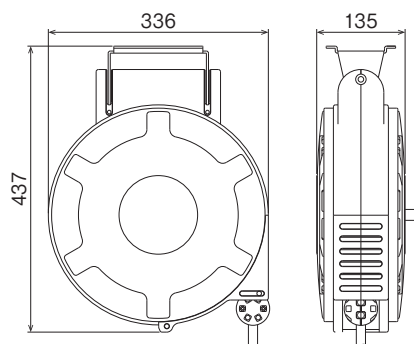
コードマックL CLD型
