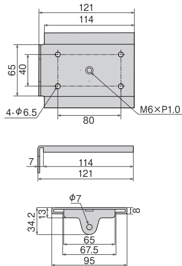
●コードマックII用 (CDS II型)
