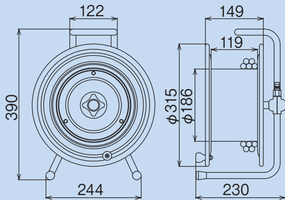
AC型
