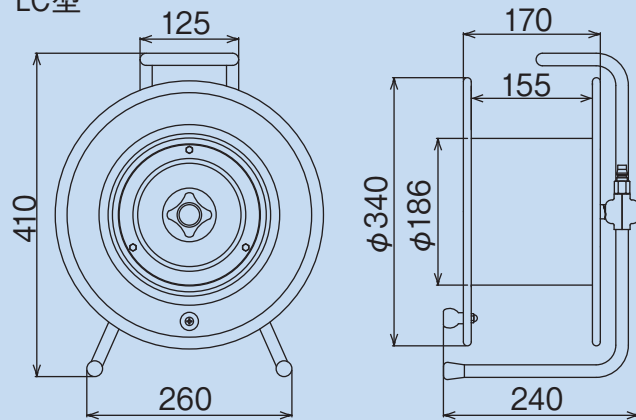
LC型
