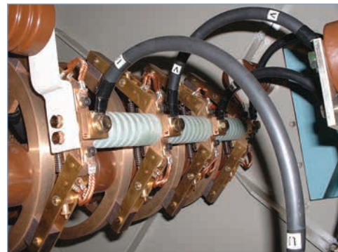
CAHS型内部(スリッピング部)
